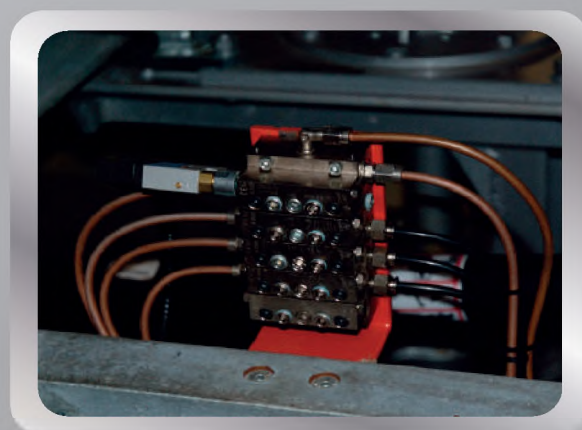
Централизованная система смазки
